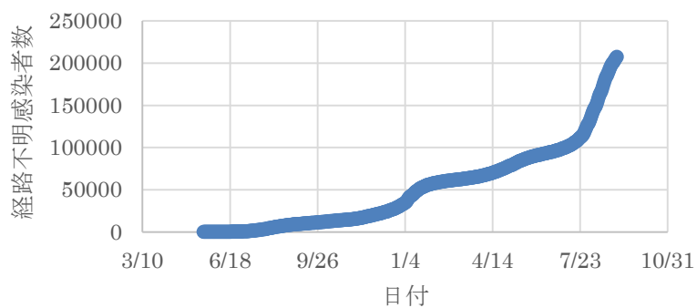
経路不明感染者累積数（東京都）
