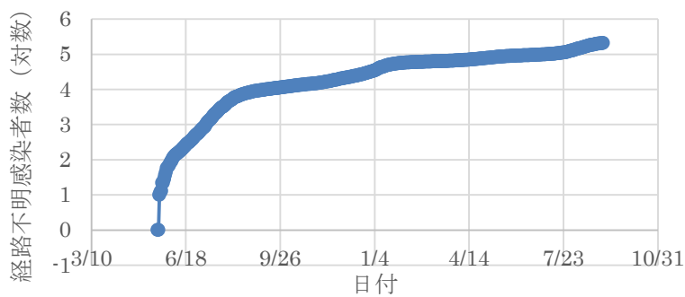
経路不明感染者累積数の対数（都）
